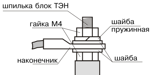
Рис.5 Присоединение проводов к выводам блок-ТЭН
