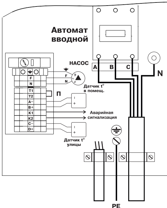
Рис.3 Схема подключения электроводонагревателя
