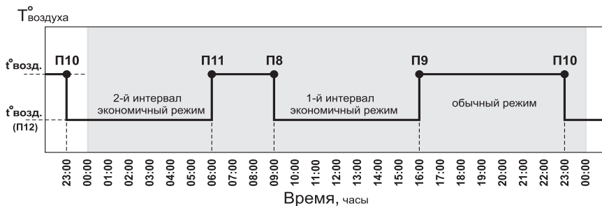
Рис.6 График температуры воздуха в помещении для Режим 1
